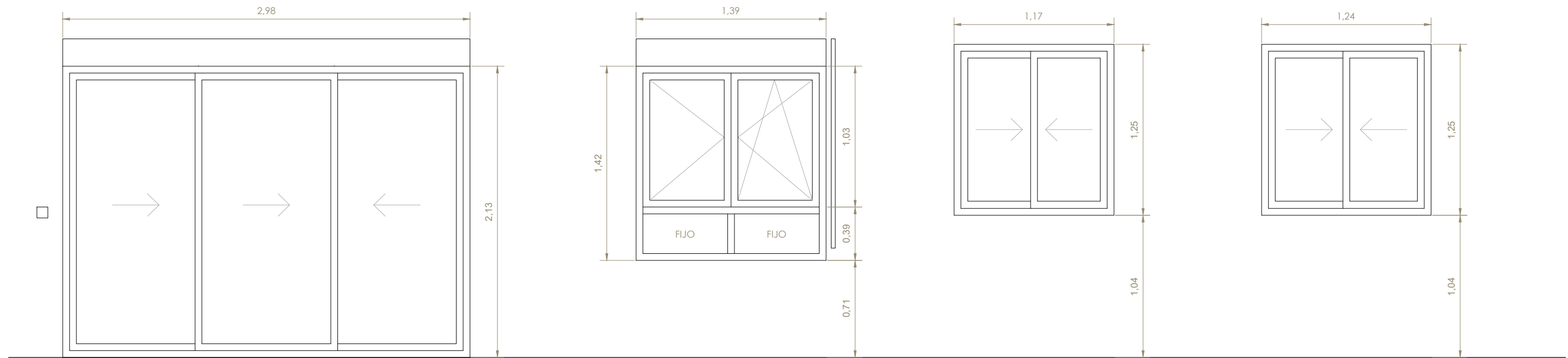
V01 3 hojas correderas Bicolor Cobre ext/Blanco int Persiana mecanismo eléctrico Nudo central minimalista
